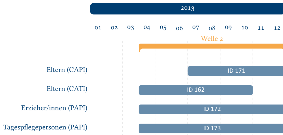
Abbildung 2: Befragungsverlauf für die Startkohorte 1 und IDs der eingesetzten Erhebungsinstrumente in Welle 2
